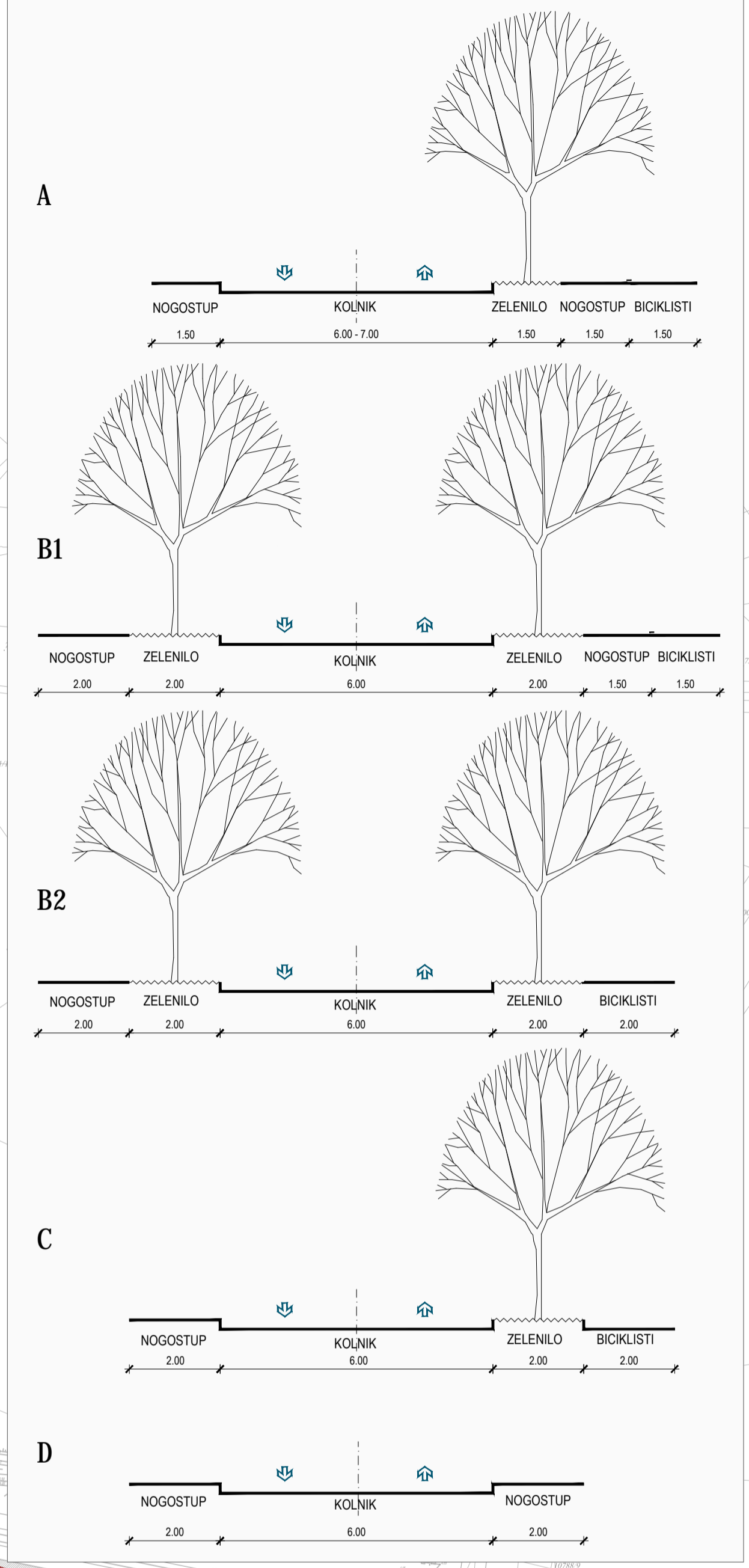
KARAKTERISTIČNI PRESJECI PROMETNICA
